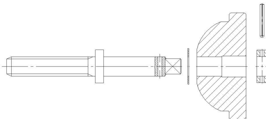
Bild 1 (nach Zeichnung 4.130881)
